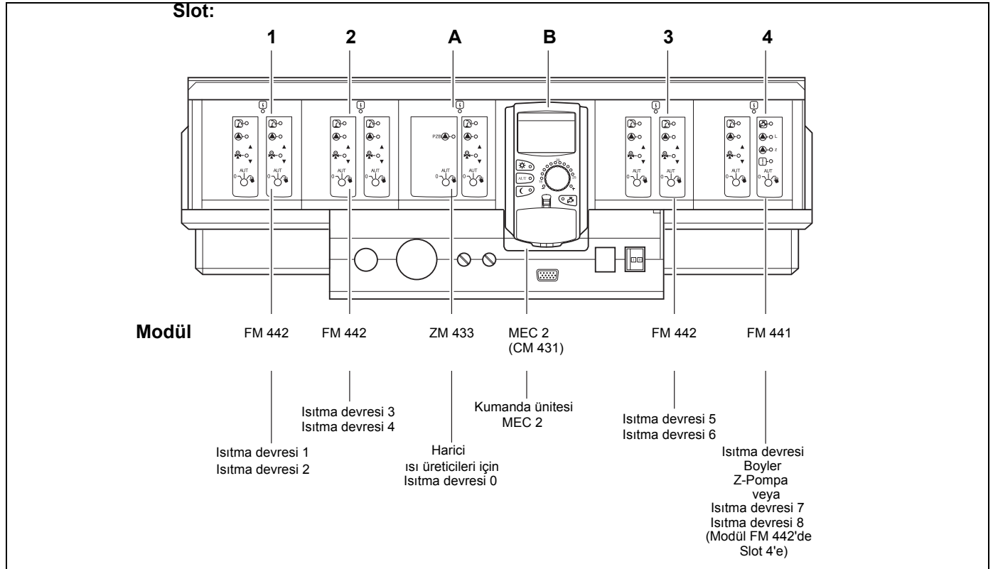
Şekil 5 Modül donanımı (mümkün olan tam donanım)
