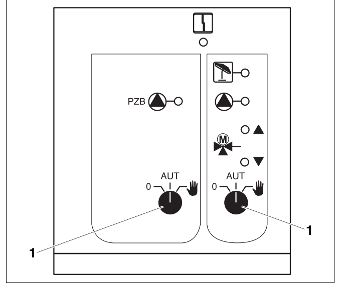
Şekil 8 Manuel kumanda şalteri, örn. merkezi modül ZM 433 üzerinde
