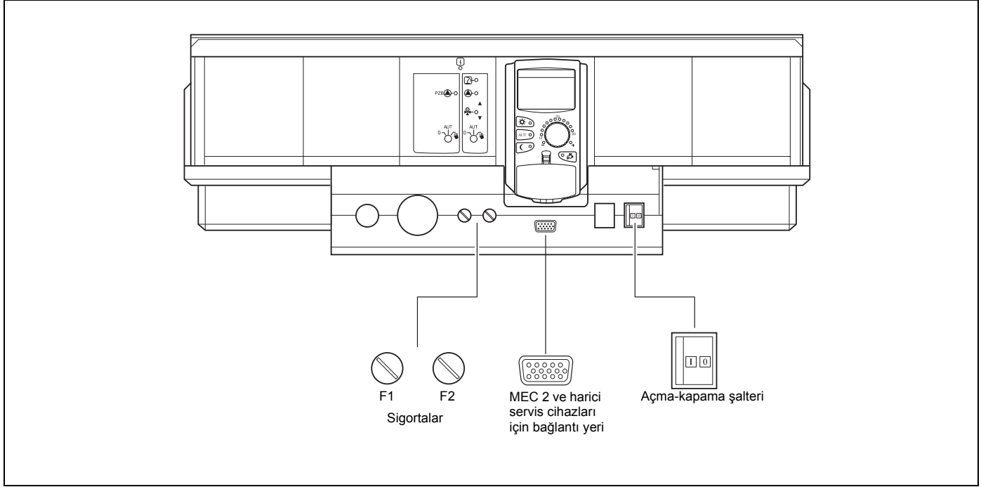
Şekil 4 Kullanma elemanları (temel donanım)
